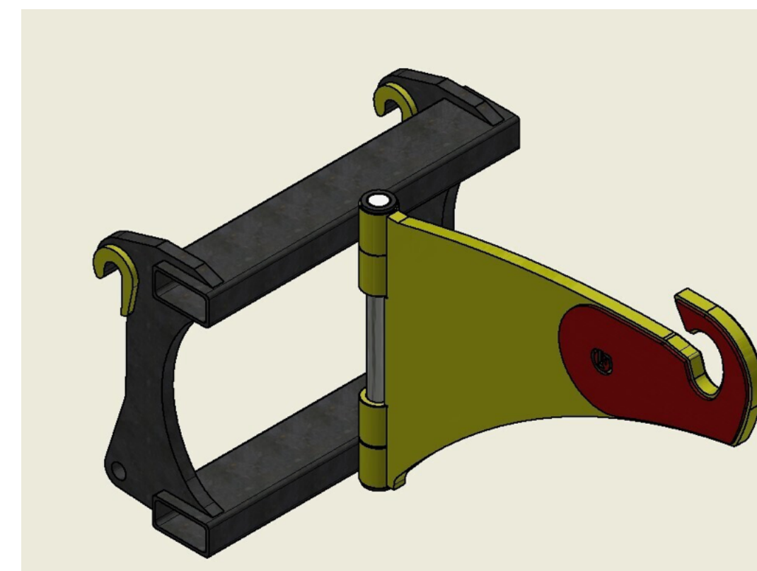
Containerhaak Crochet d'attelage
